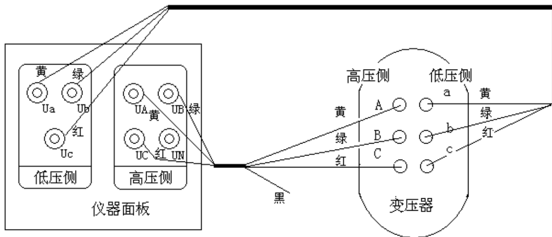
图十四、三相变压器的测试接线
