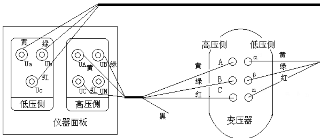
图十七、斯科特型变的测试接线
