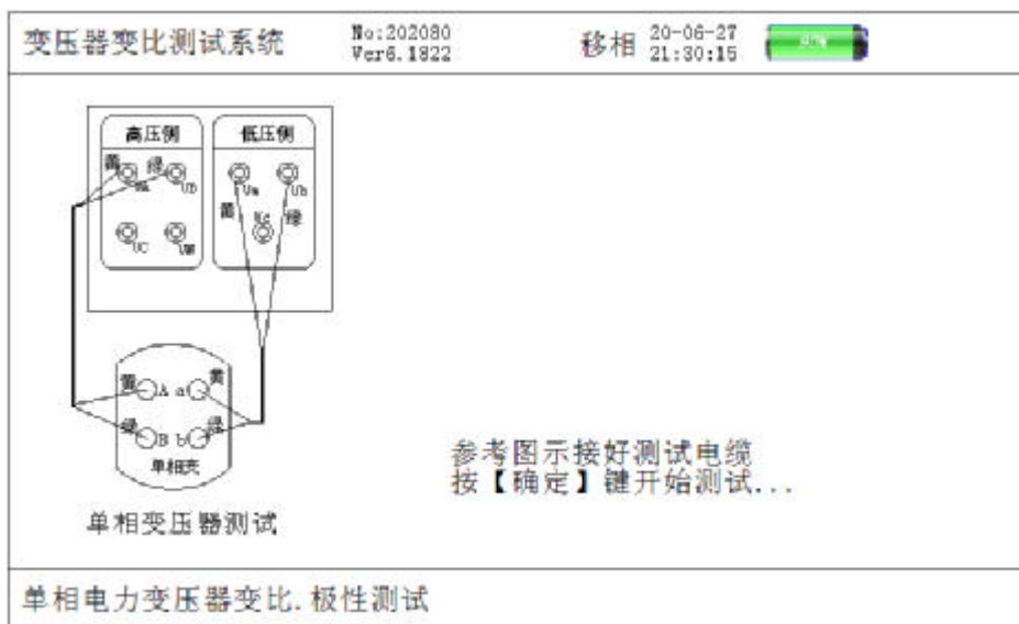
图九、单相变压器测试接线提示屏
