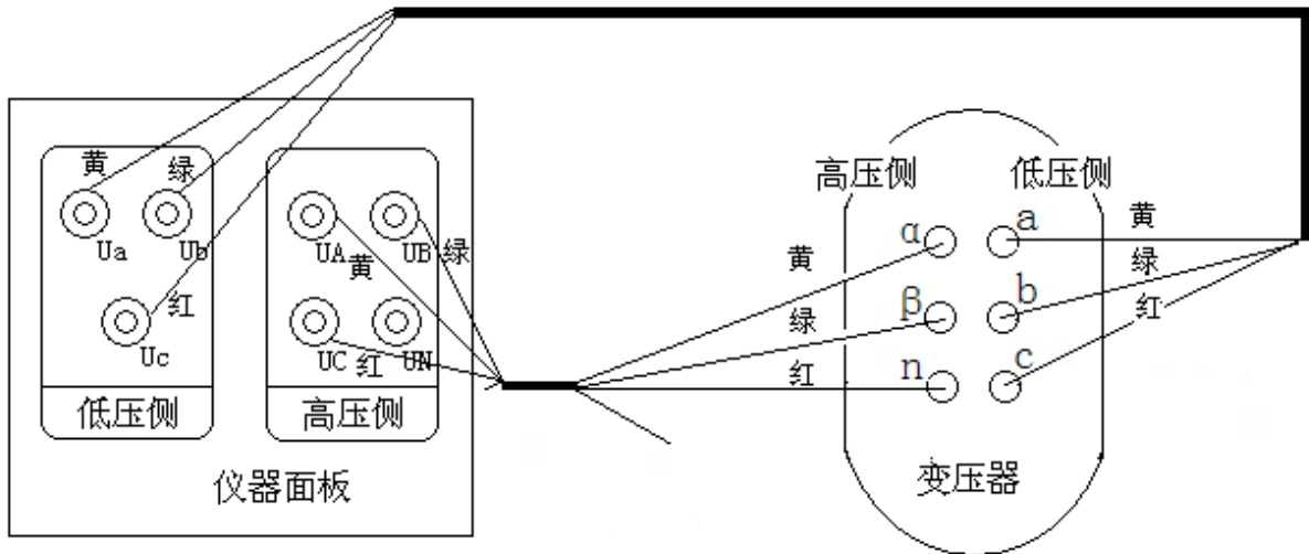
图十八、逆斯科特变压器的测试接线
