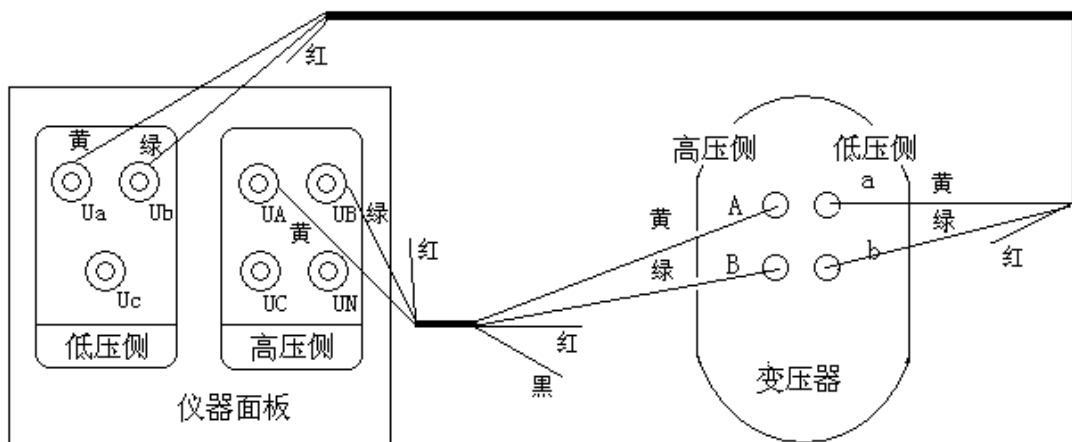
图十五、单相变压器的测试接线
