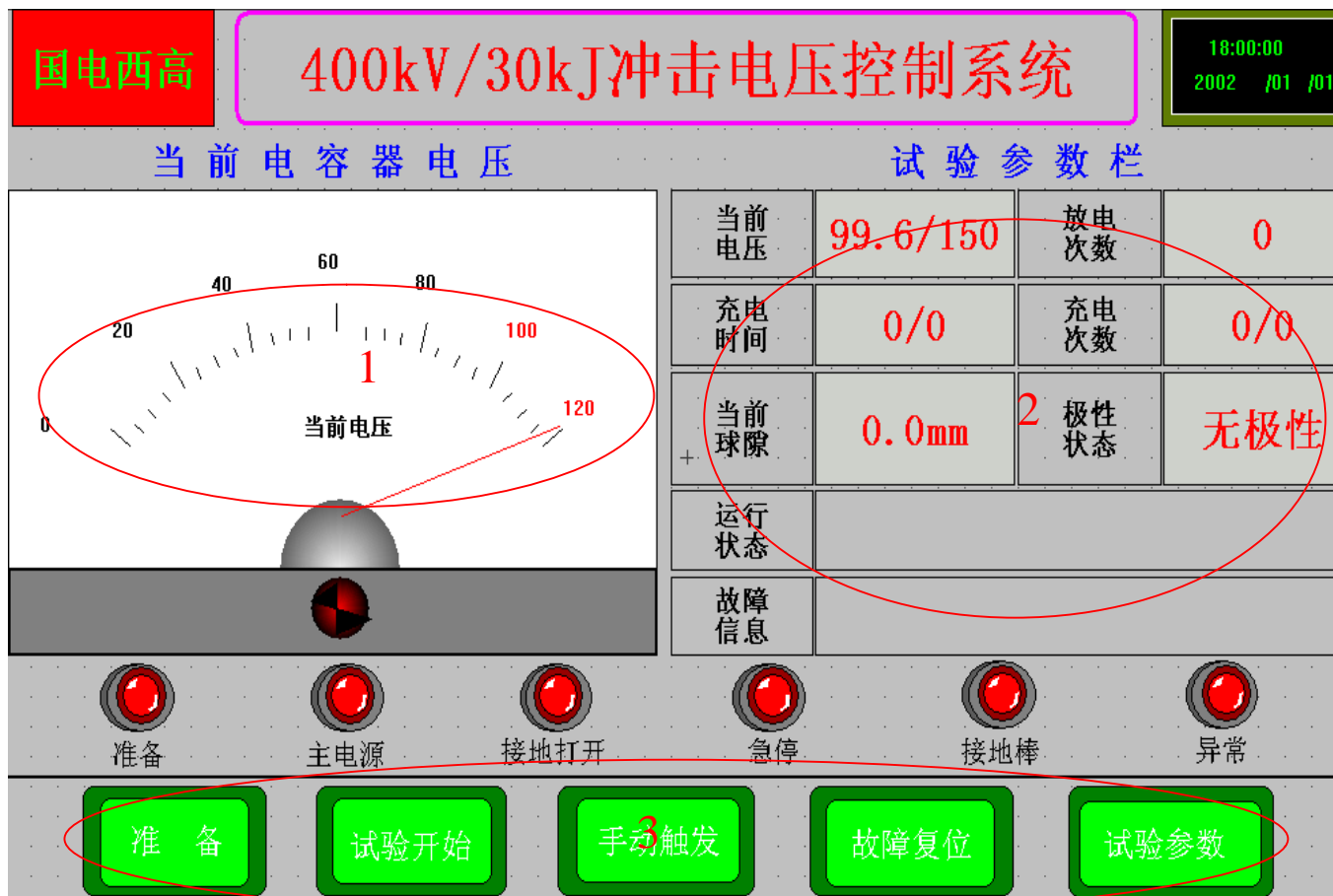
图 7-2 主控界面
