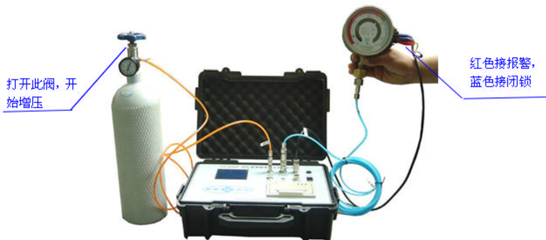
(校验密度继电器整体连接图)
