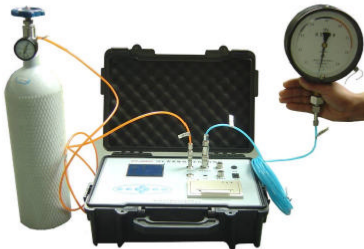
(压力表检测连接示意图)
