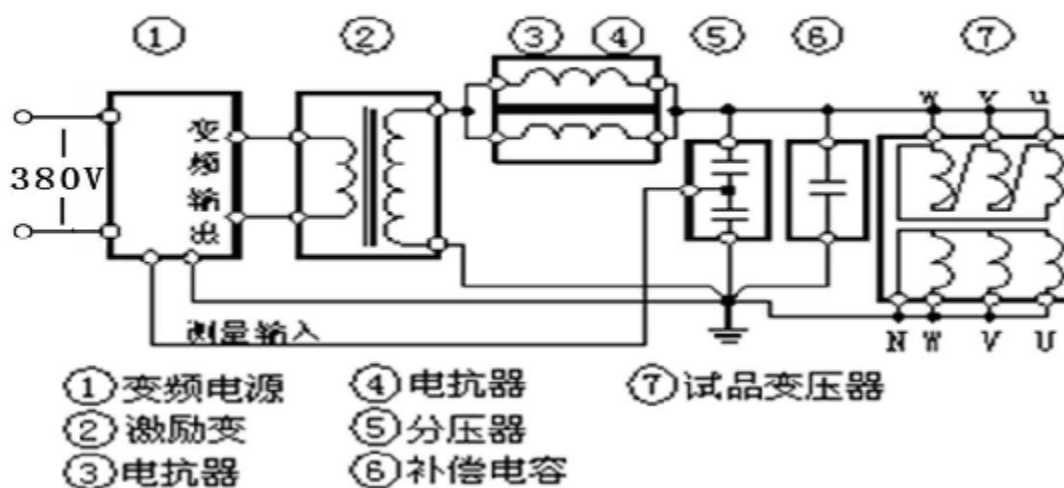
变压器耐压试验接线图
