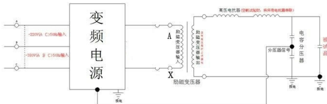
调频谐振试验接线示意图
