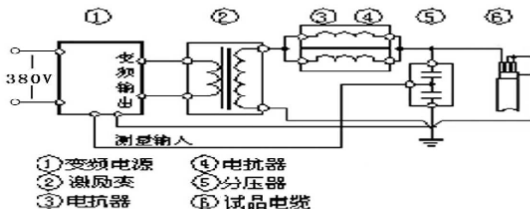
电缆耐压试验接线图
