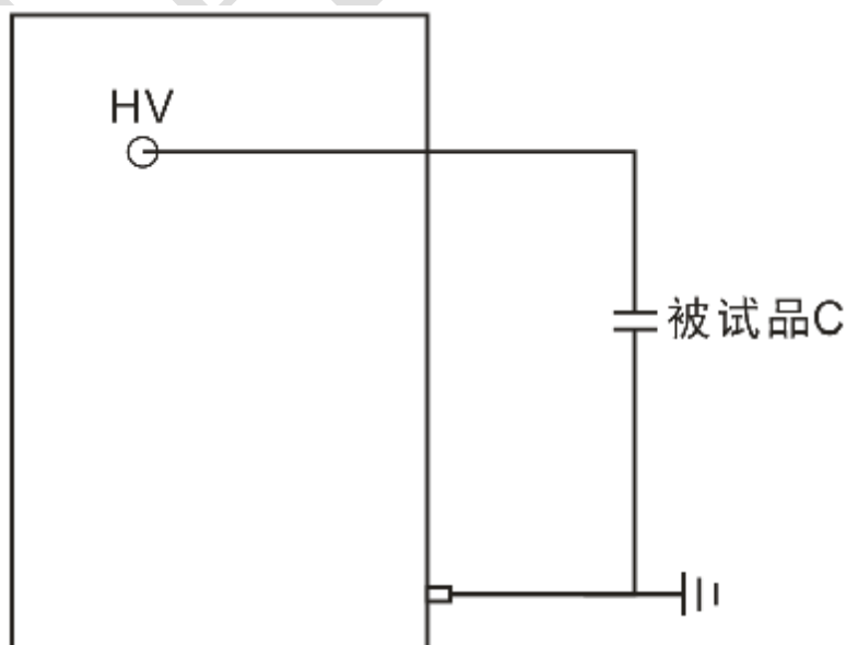
被试验接线示意图
